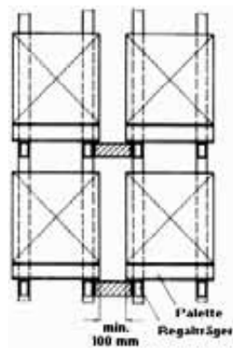
Abb. 8b: Sicherheitsabstand
