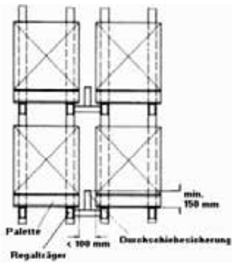
Abb. 8a: Durchschiebesicherung
